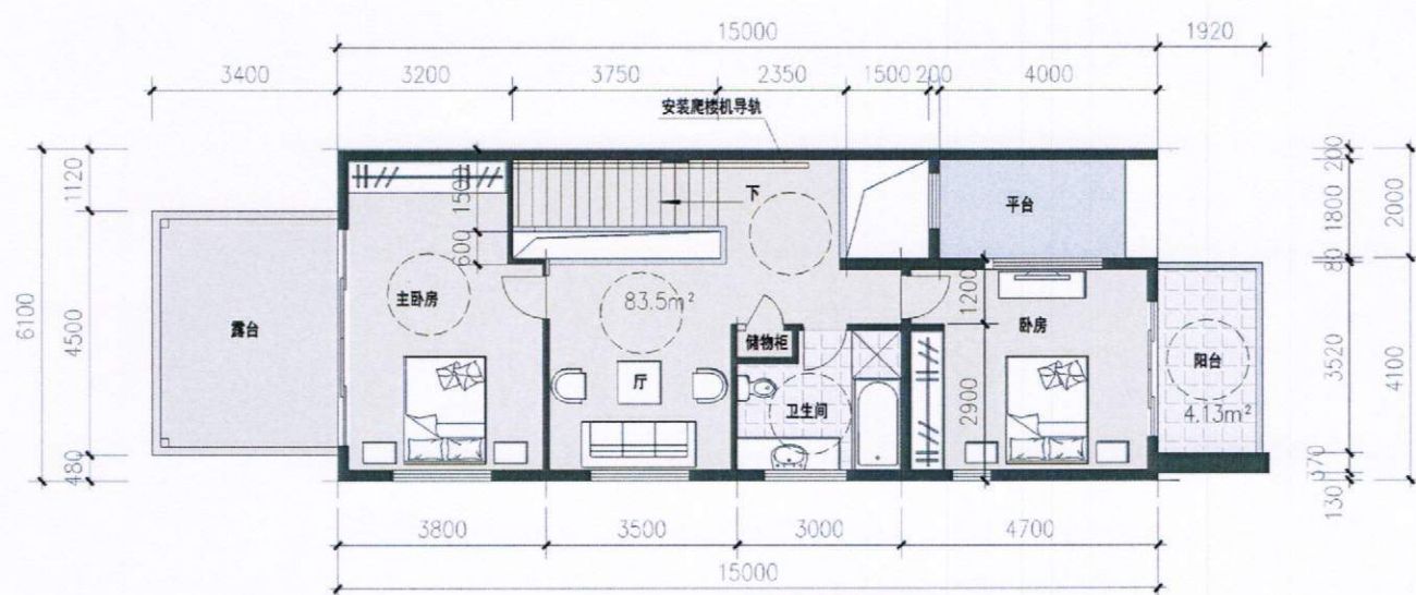
二层平面图
